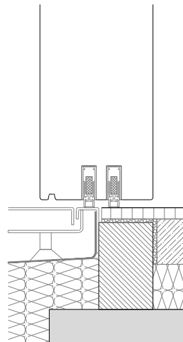
Streiftür mit Draingerost (nicht geeignet für stark bewitterte Bereiche)
