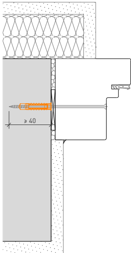
Leibungsmontage
