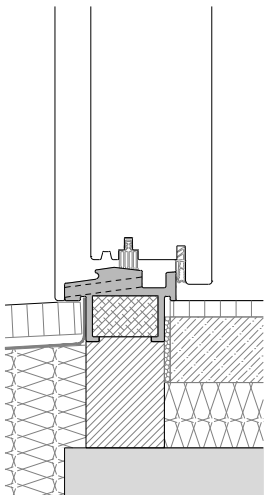
GFK Schwelle AG 168 1.02
