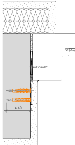
Leibungsmontage mit Ankerblech
