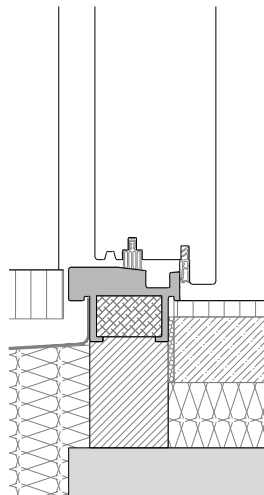
GFK Schwelle AG 168 1.01
