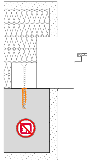
Blendrahmenmontage
