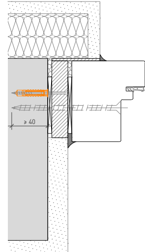
Leibungsmontage mit Blindstock
